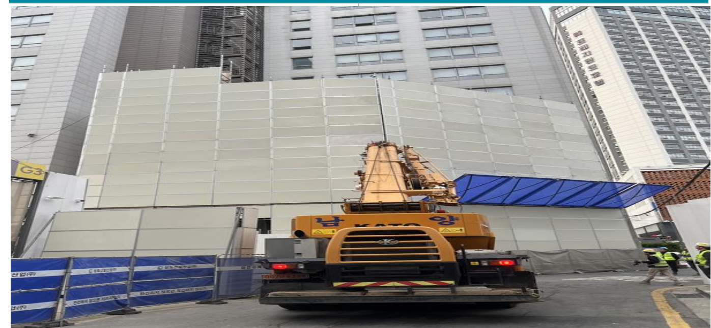
서울 을지로 제주본가 철거 및 시스템 매직판넬 시공 공사 (CJ)
