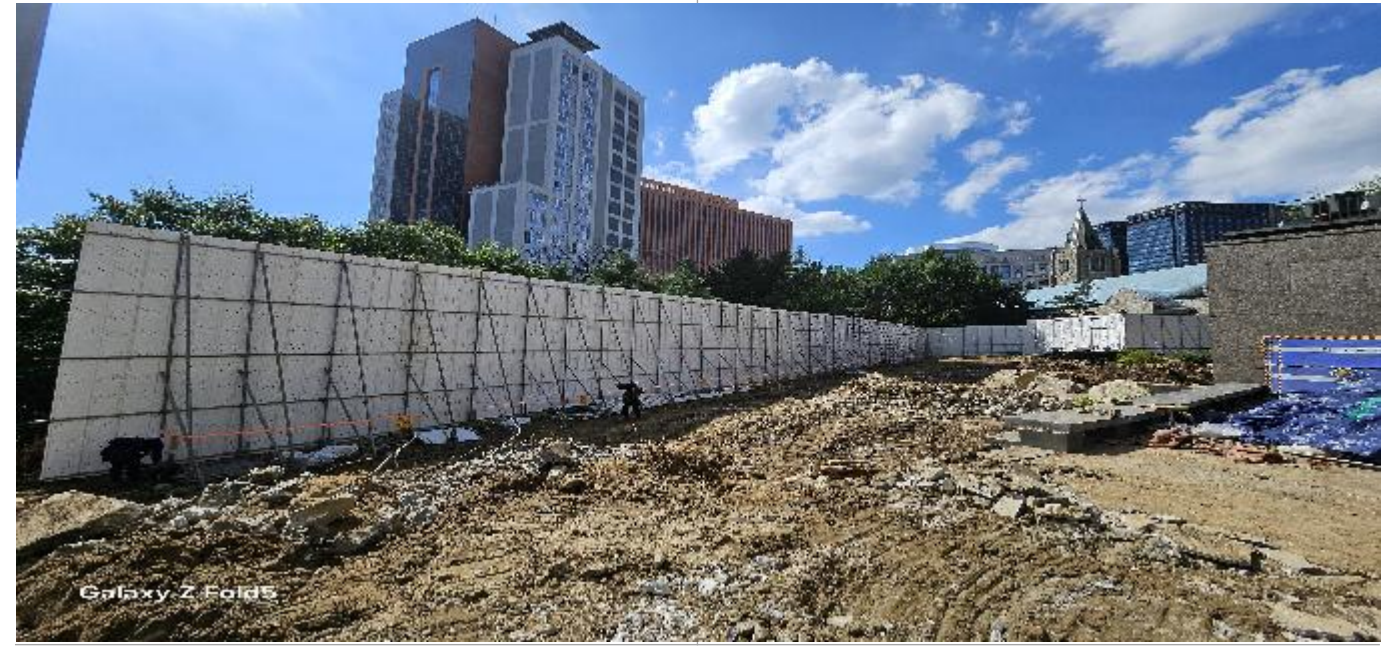
서울 방배동 rpp공사
